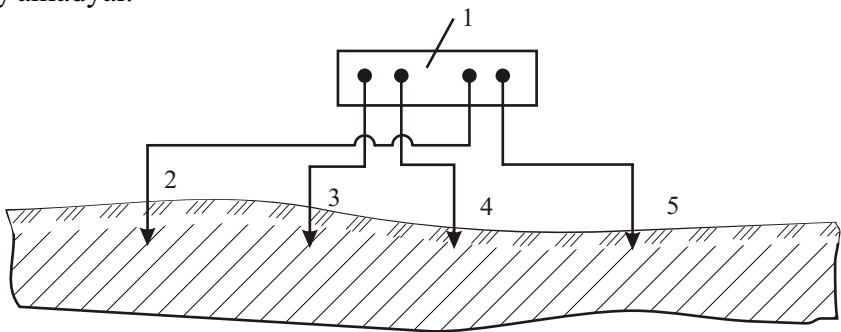
32-nji surat. Dag jynslarynyň elektrik kesme usuly bilen öwrenilişi: 1 – abzal; 2-5 – elektrodlar
