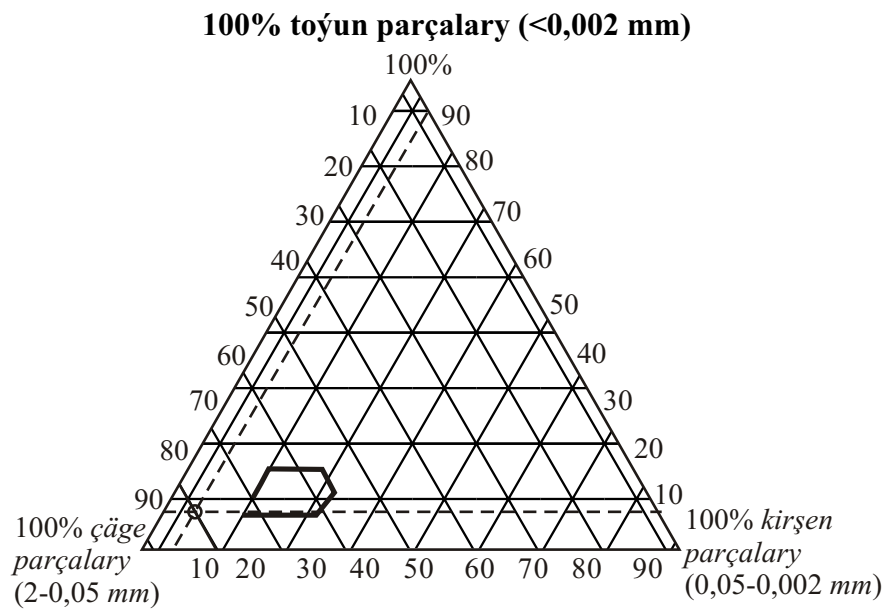
3-nji surat. Teýgumlaryň zire düzümini şekillendirýän üçburçly çyzgy
