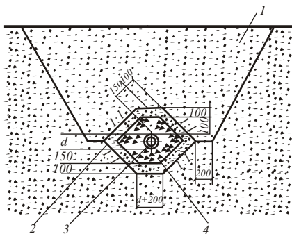
17-nji surat. Kämil däl kysymly turbaly zeýkeş.
