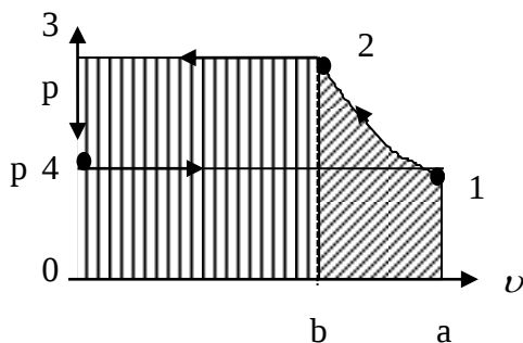
5.2 –nji surat. Gazyň ululyklarynyň p-\nu diagrammasy
