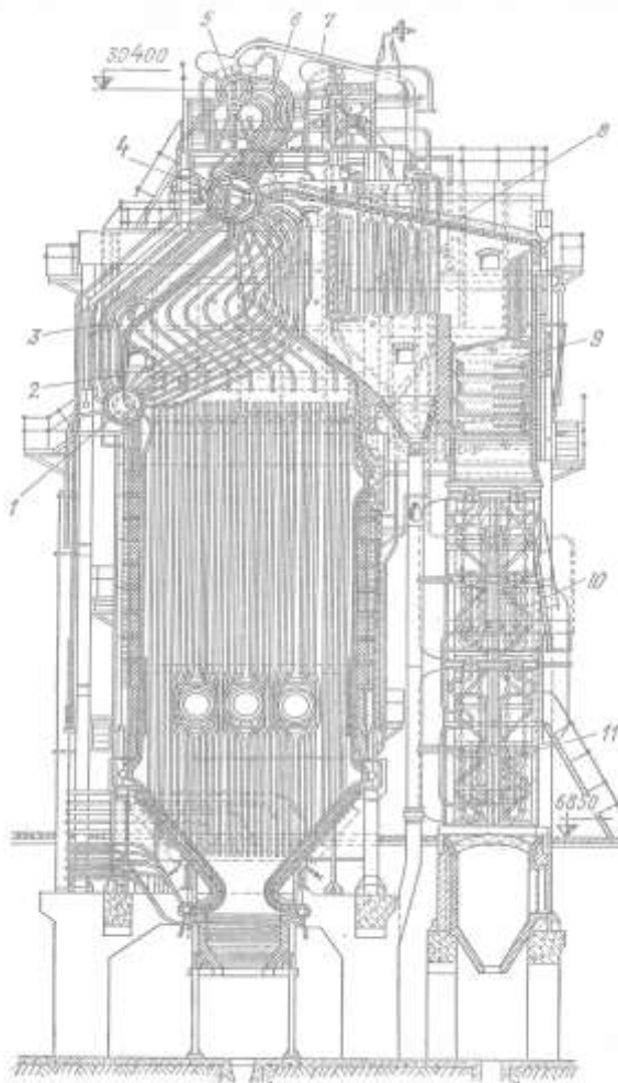
23.7-nji surat. SKTI-TKZ iki barabanly gazanda gurnalan toz-an – kömür kameraly ojak.1-aşaky baraban, 2-gazan turba dessesi, 3-aşak goýberiji turbalar, 4-ýokarky baraban, 5-gury bug alyjy, 6-bugy täzeden goýberiji turbalar, 7-doýgun buguň bug geçirijisi, 8-bugy aşa gyzdyryjy, 9-suw ekonomayzeri, 10-howa gyzdyryjy, 11-üfleýji enjamlaryň birikmeleri
