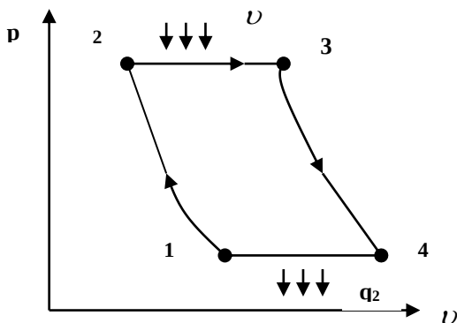
7.4-nji surat. Aýlawyň p-v diagrammasy
