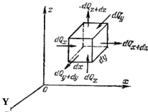
12.2-nji surat. Ýylylyk geçirijiligiň differensial deňlemesiniň getirilip çykarylyşy.
