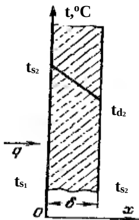
18.1-nji surat. Diwaryň galyňlygy boýunça temperaturanyň üýtgeşi
