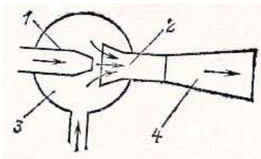
11.5-nji surat. Ežektor abzalynyň shemasy
