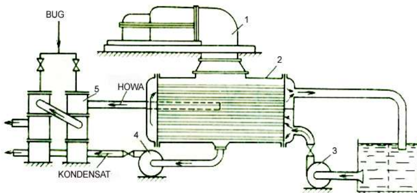
25.8-nji surat. Kondensirleýän desganyň prinsipial shemasy 1-bug turbina; 2-kondensator; 3-aýlanyşyk nasos; 4-kondensat nasosy; 5-bug ežektory
