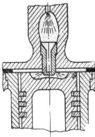
27.4-nji surat. Bölünmedik ýandyrys kameranyň prinsipial shemasy
