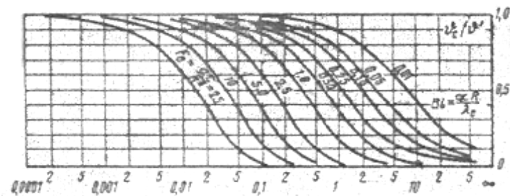
14.6-njy surat. Uzynlygy tükeniksiz silindr üçin
