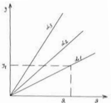
20.1-nji surat. Tüsse gazynyň temperaturasyna we howanyň artykmaçlyk koeffisiýentine baglylykda entalpiýasy
