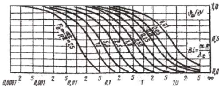
14.9-nji surat. Şar üçin \vartheta_c / \vartheta' = \Phi_c(Bi, Fo) baglylyk
