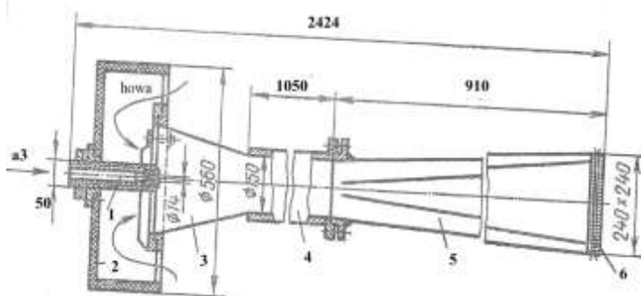
23.12-nji surat. Inžener Kazansewiň konstruksiýaly IGK-250 injeksion gorelkasy:
