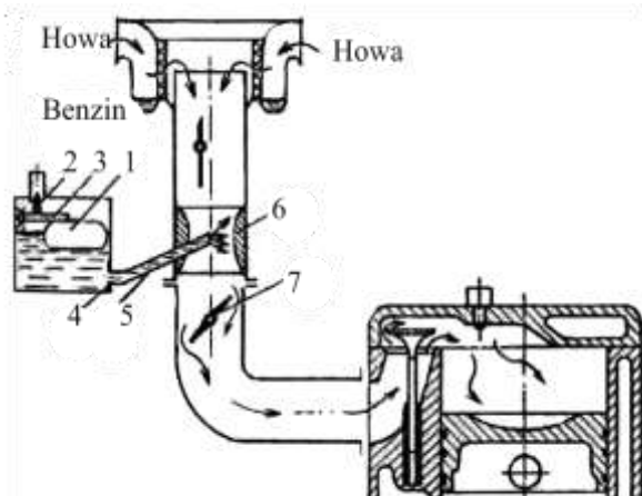
27.2-nji surat. Ýönekeý karbýuratorýň prinsipial shemasy
