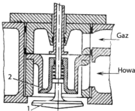
27.5-nji surat. Gazgaryjy sorujy klapnan
